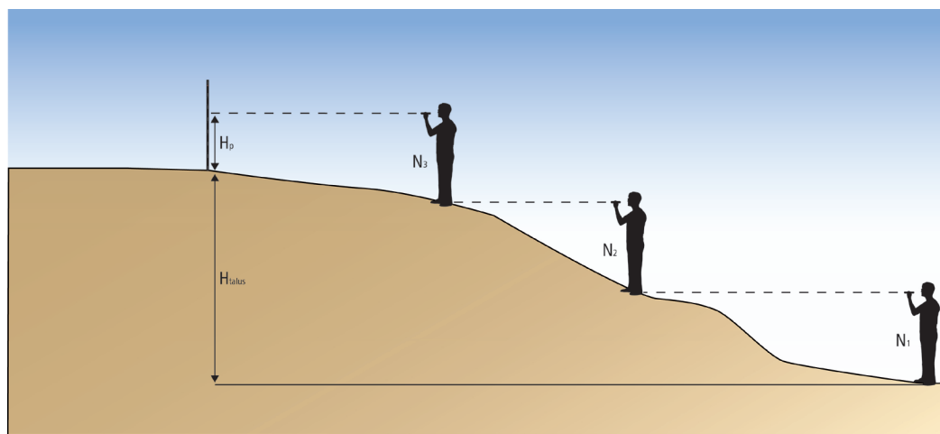
Figure 3 | Détermination de la hauteur d'un talus
