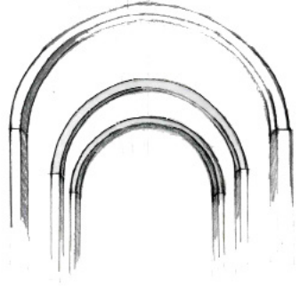
Voûte en berceau
