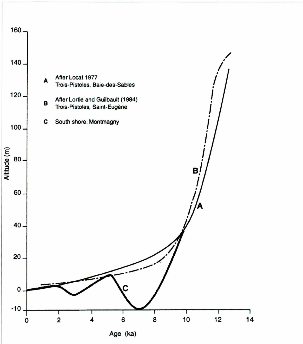
Figure 2 : Courbe d'émersion des terres dans l'estuaire du Saint-Laurent (source : Dionne 1988: 241).
