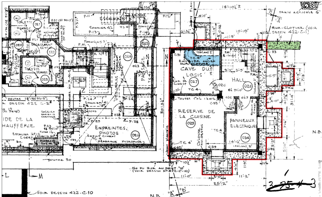
Figure 6.9 Détail du sous-sol du nouveau logis du géôlier dans le plan de restauration de 1959 (Cyr). La section de l'ancien mur de la cour qu'il est prévu d'enlever est rehaussé en bleu. L'emplacement du nouveau mur est rehaussé en vert.
