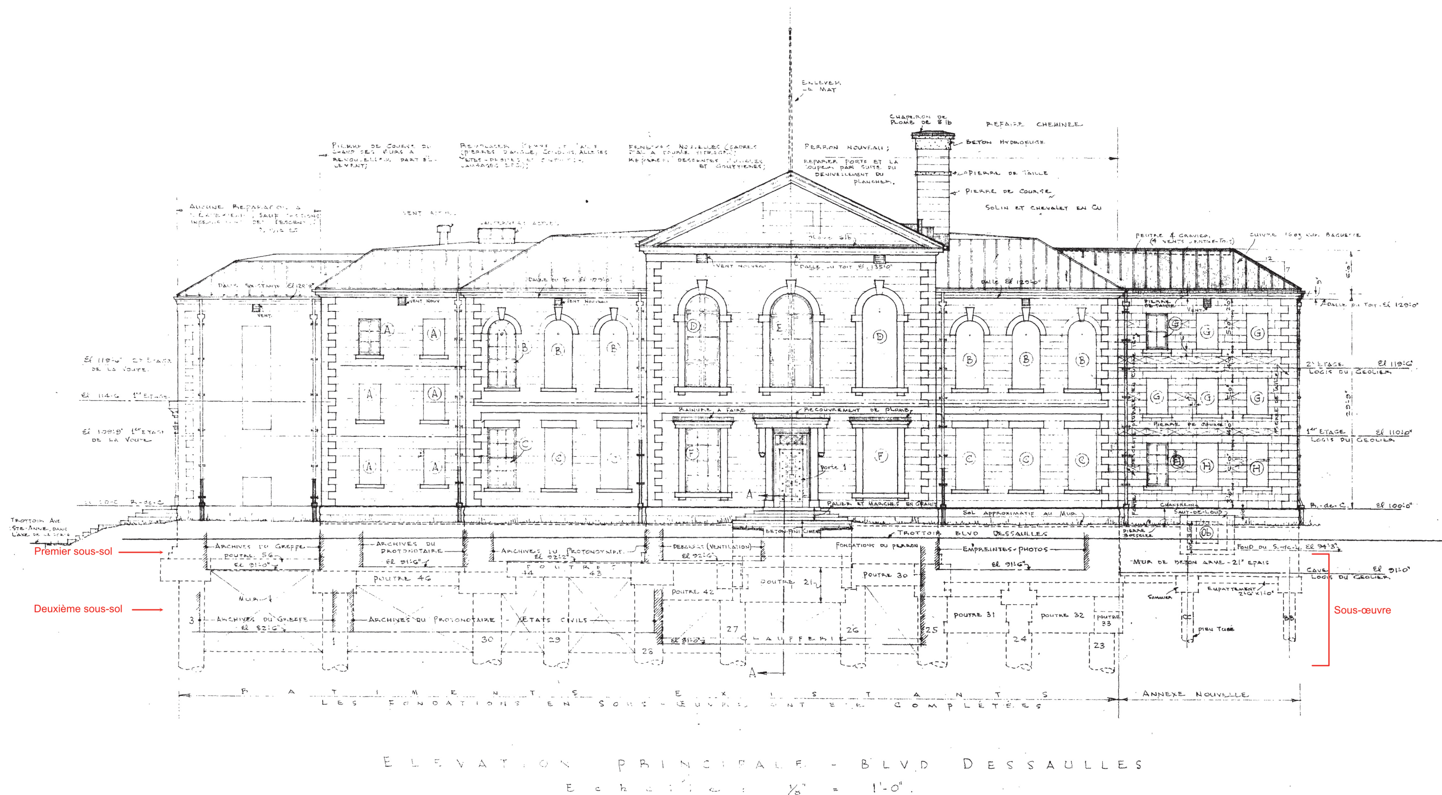
Figure 5.16 Détail du plan de restauration et agrandissement du palais de justice et prison de Saint-Hyacinthe, 1959 (Cyr). On voit ici l'élévation de la façade du bâtiment. Le sous-cœuvre en béton est représenté par les lignes tiretées.
