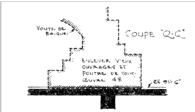
Figure 6.7 Coupe du mur nord de l'ancienne voûte du protonotaire telle que représentée dans le plan de restauration de 1959 (Cyr)
