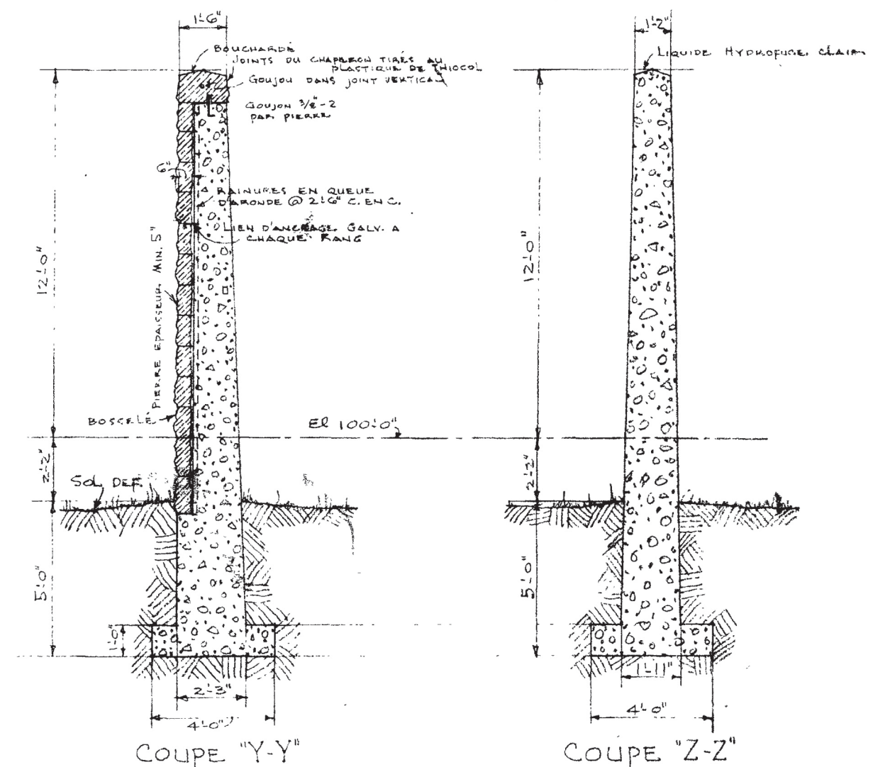
Figure 5.20 Détail du plan de restauration et agrandissement du palais de justice et prison de Saint-Hyacinthe, 1959 (Cyr). Coupes de l'élévation du nouveau mur de la cour en béton
