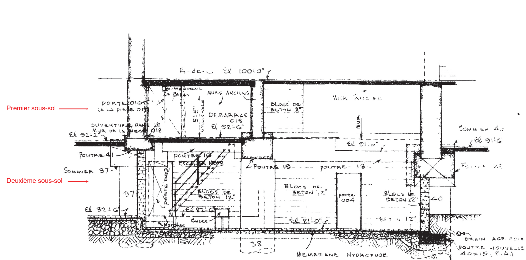
Figure 5.19 Détail du plan de restauration et agrandissement du palais de justice et prison de Saint-Hyacinthe, 1959 (Cyr). Aperçu de l'élévation des sous-sols avec les parties anciennes et en sous-œuvre.
