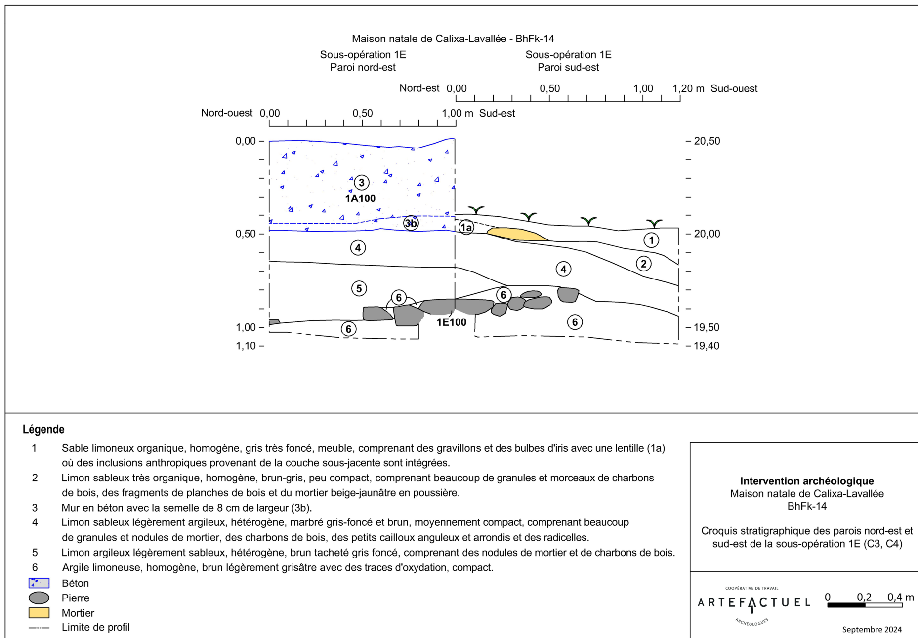
Figure 4.10 Coupe stratigraphique des parois nord-est et sud-est de la sous-opération 1E. Infographie : Archéo-CAD.
