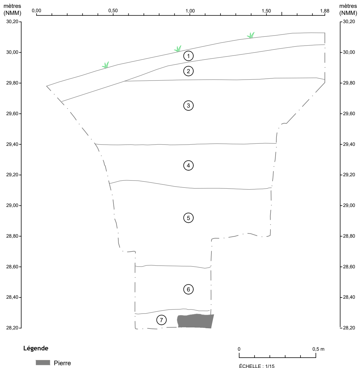
Figure 18 - BjFj-232 – Sous-opération 2F – Coupe C4, paroi sud-est
