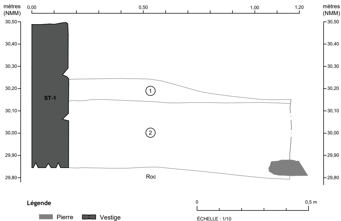
Figure 17 - BjFj-232 – Sous-opération 2B – Coupe C2, paroi nord-ouest
