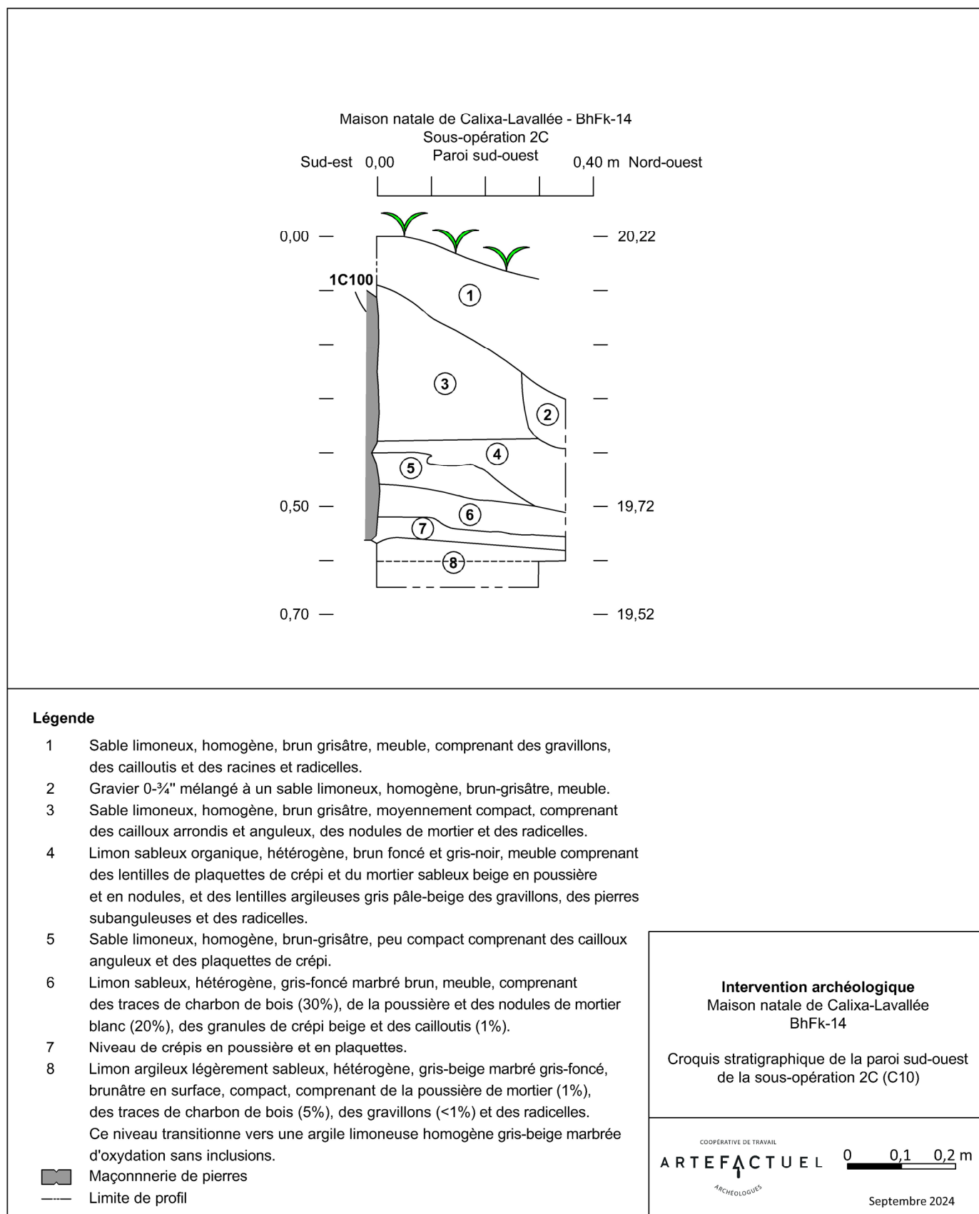
Figure 4.7 Coupe stratigraphique de la paroi sud-ouest de la sous-opération 2C. Infographie : Archéo-CAD.
