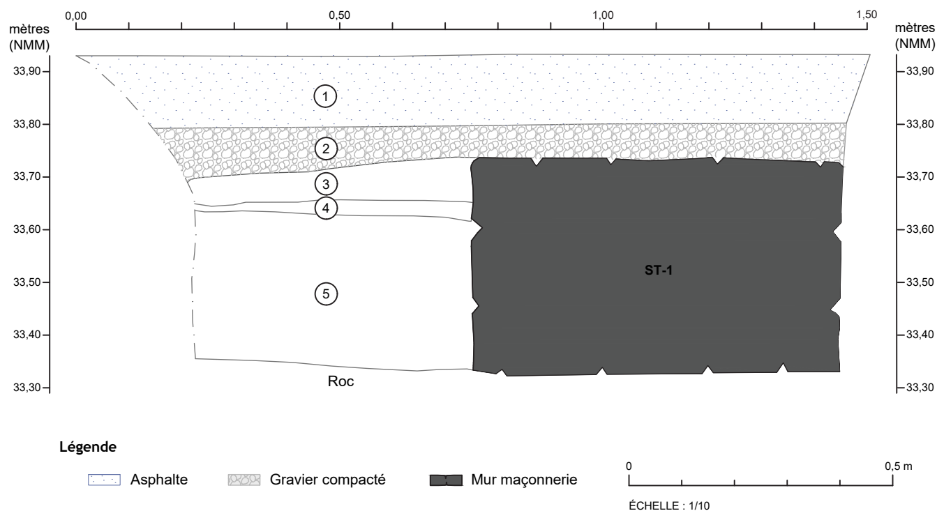
Figure 13 - BjFj-231 – Sous-opération 2A – Coupe C1, paroi nord-ouest
