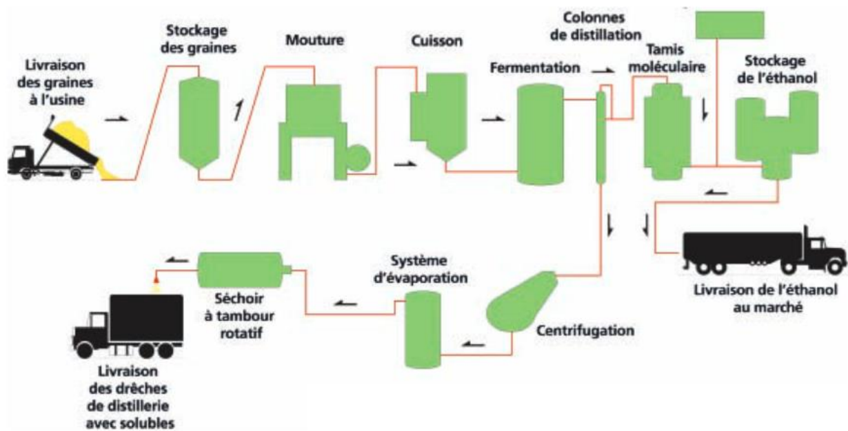
Figure 1.1 : Procédé de production d'éthanol de première génération (tiré d'AgriRéseau, 2007)
