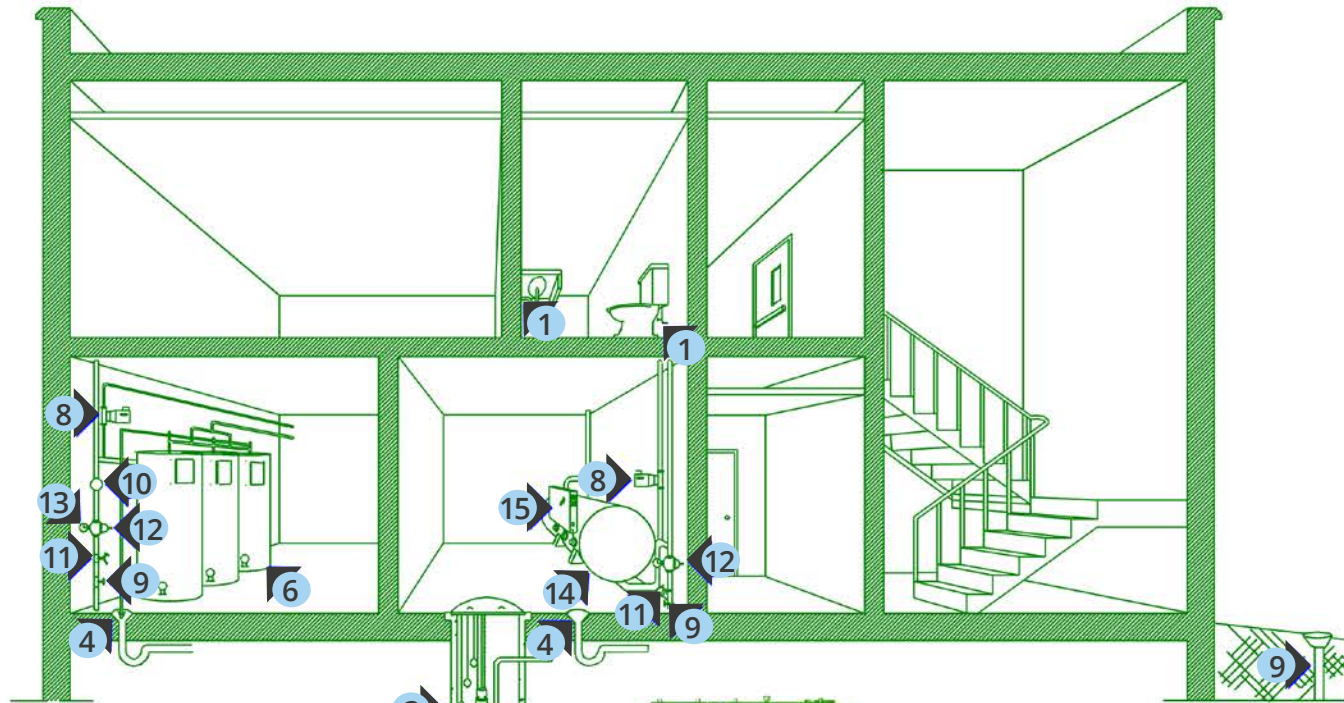
12 Réducteur de pression
