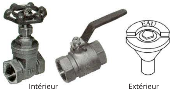
9 Robinets principaux d'arrêt d'eau
