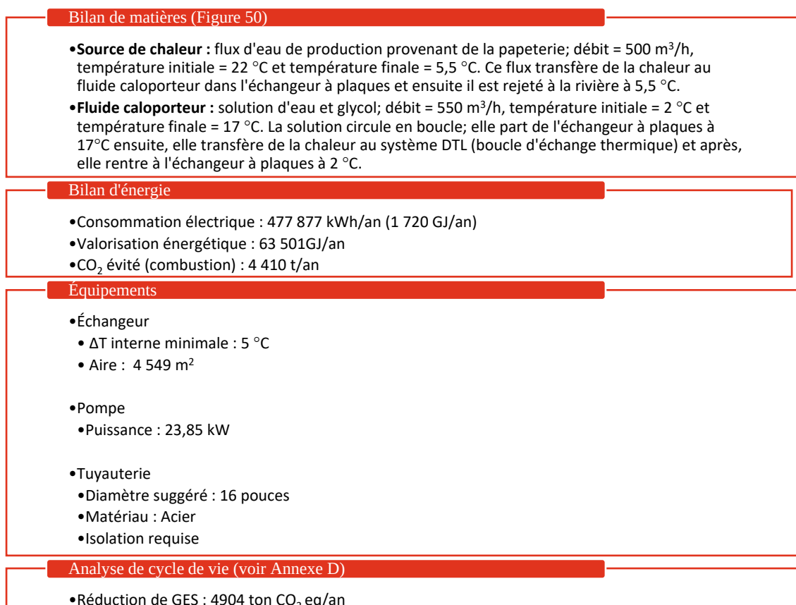
Figure 51 : Bilans de matière et d'énergie de la valorisation thermique des gaz de pyrolyse de Xylo-Carbone
