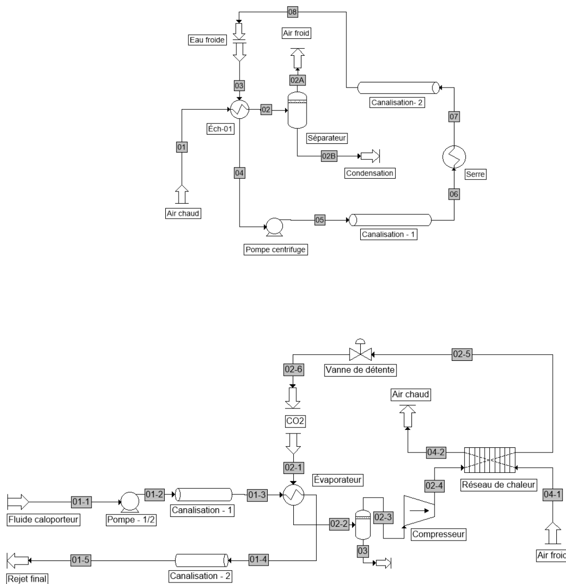
Figure 31 : Exemple de schémas de principe pour la valorisation énergétique sur Prosim Plus
