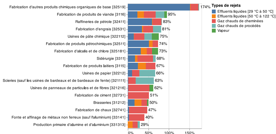
Figure 3 : Graphique présentant les ratios des rejets thermiques en fonction de la consommation énergétique provenant de Stricker Associates Inc. (2007)
