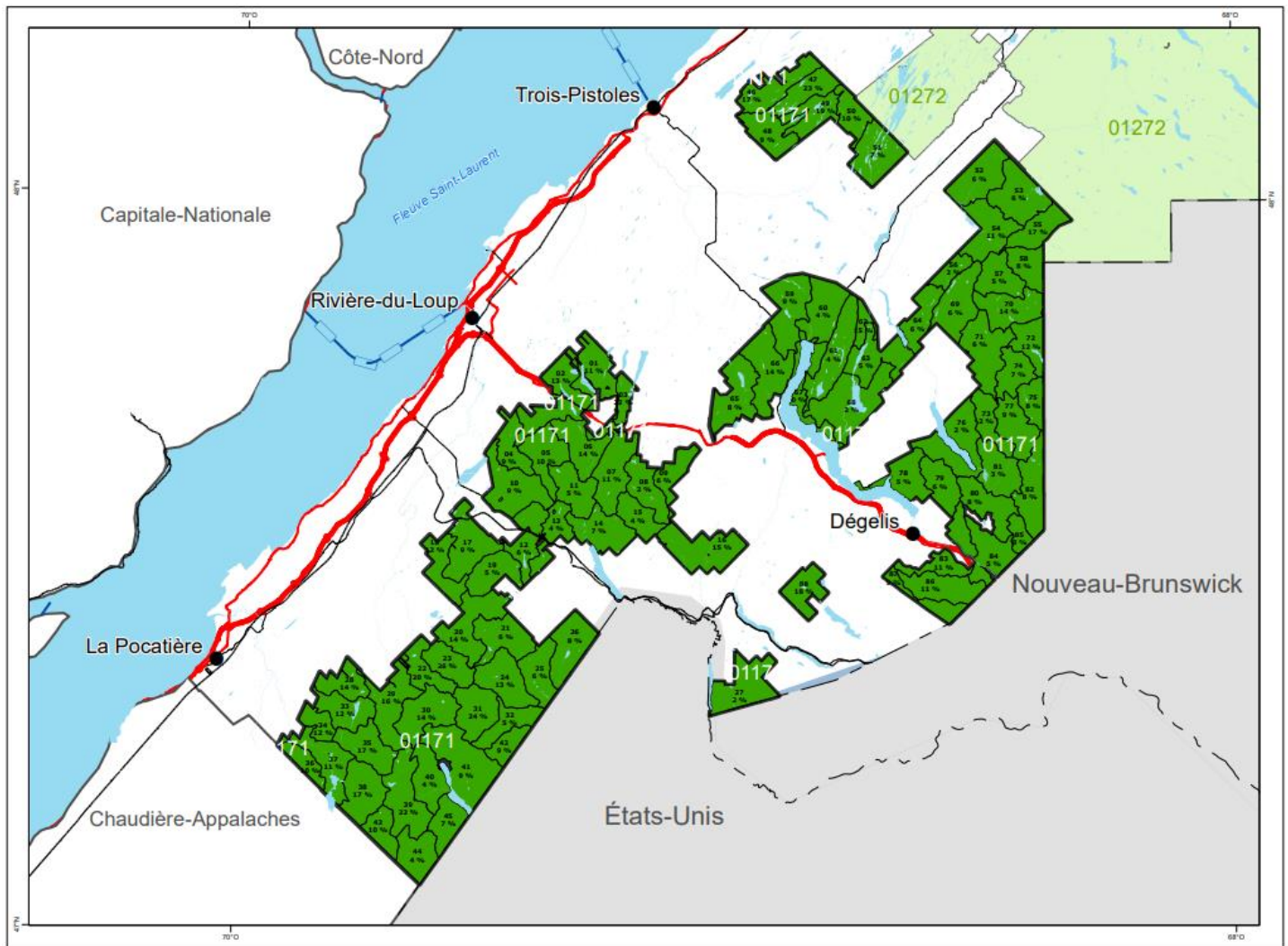
Figure 12 Proportion et degré d'altération des forêts de moins de 20 ans dans l'UA 011-71
