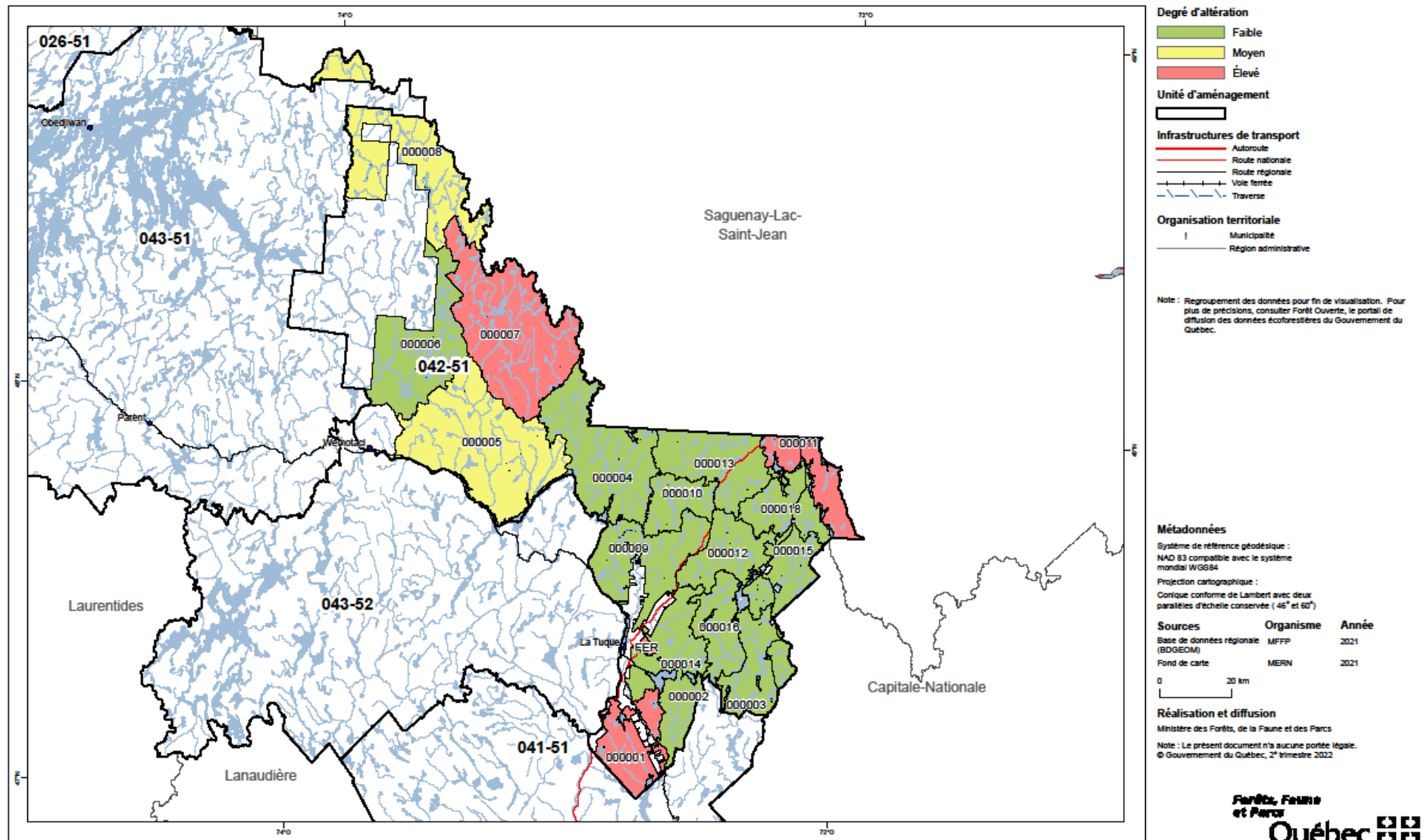
Carte 3 : Degré d'altération actuel de la structure d'âge de l'UTA au 1 er avril 2023 — UA 042-51
