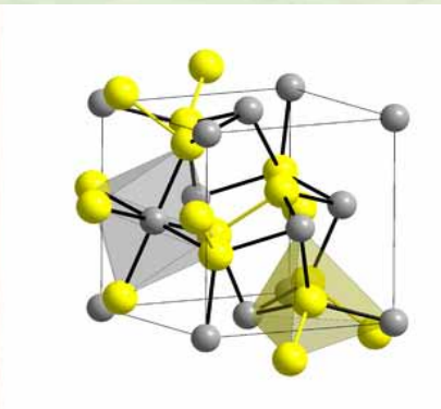
Structure cristalline de la pyrite
